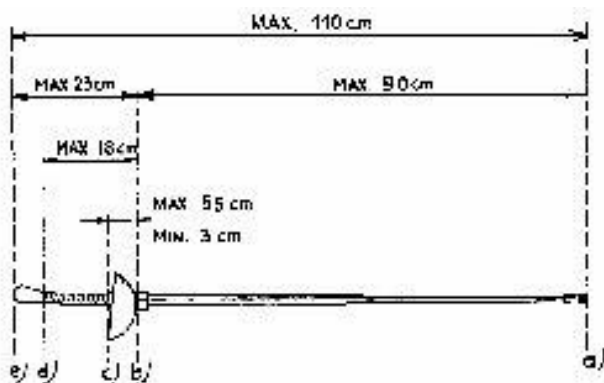
Dimensioni della spada
